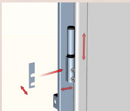
3D регулируеми панти
