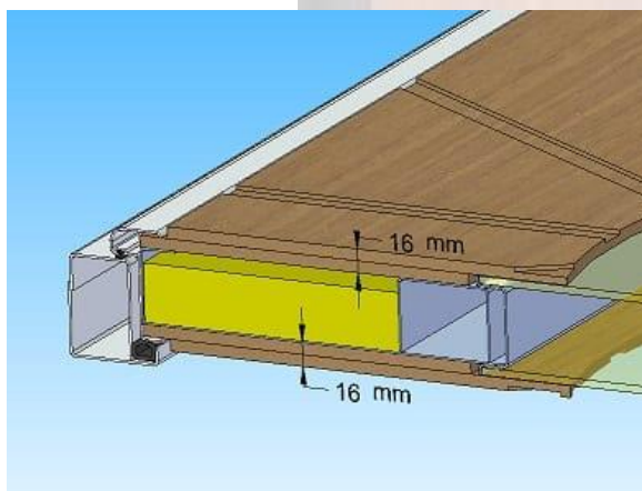
5. Разрез: xDoor Exclusive
